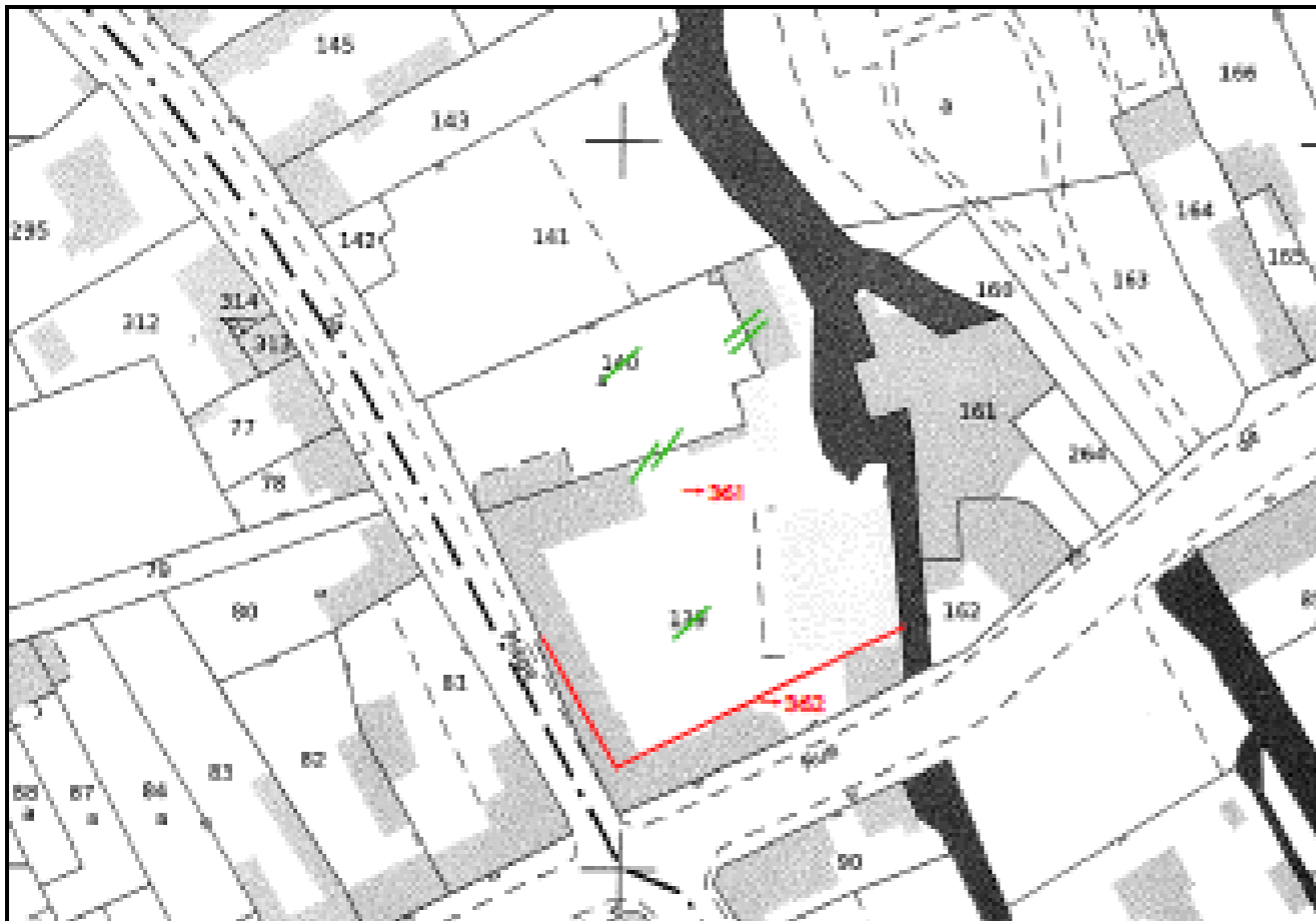
PLAN D'ENSEMBLE Echelle : 1/1000 Extrait cadastral
